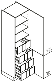
VI Larder unit ↔ 40/45/50/60 ↑ 215 ↲ 60/50/39
